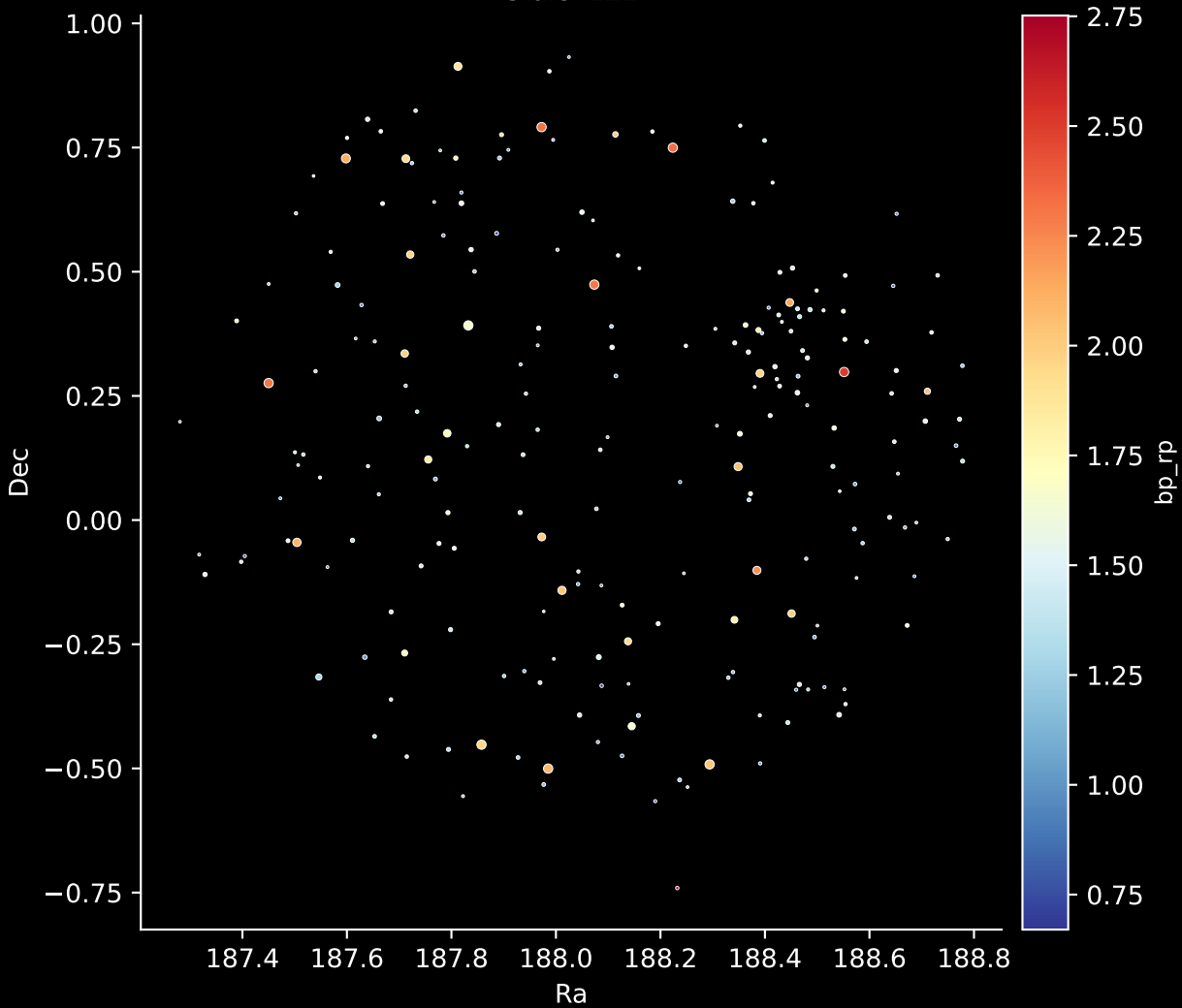
GALAH DR4 Field: [3669] Stars: 221
