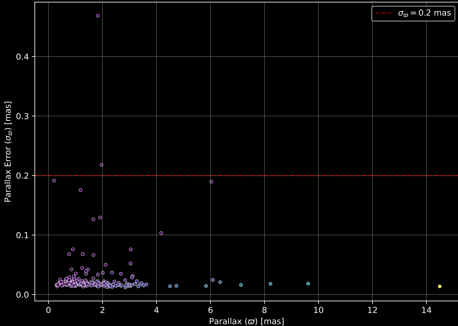
GALAH DR4 Field: [3669] Parallax Quality (n= 221)
