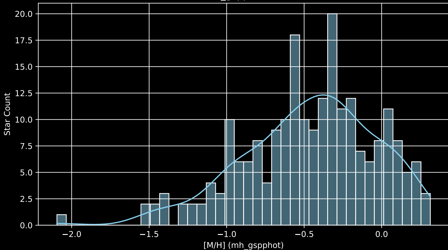
GALAH DR4 Field: [3669] [M/H] (mh_gspphot) (n= 220)
