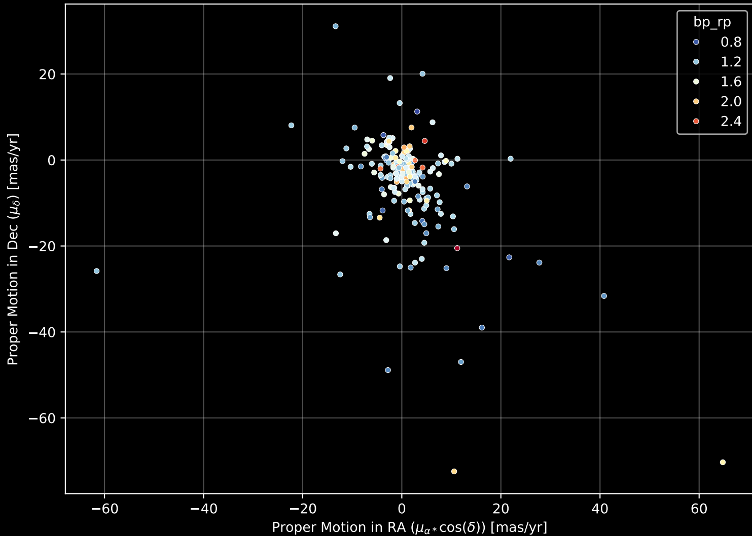
GALAH DR4 Field: [3669] Proper Motion Diagram (n= 221)
