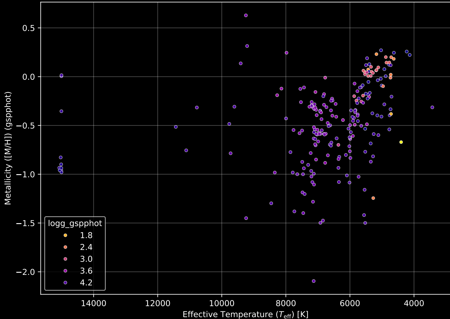
GALAH DR4 Field: [3669] Stellar Population Parameters (n= 221)
